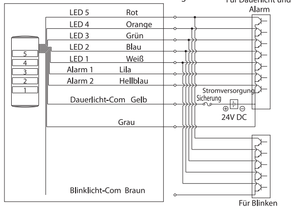
Dauerlicht oder Blinklicht mit akustischem Signal
